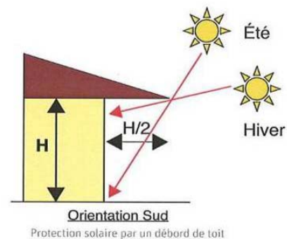
Protection solaire par un débord de toit
